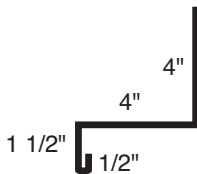
Solin finition et solin de puits de lumière #1
