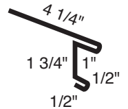
Partance pour toiture #2
