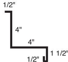
Solin finition et solin de puits de lumière #2
