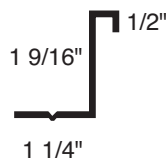
Clip de joint mécanique pour toiture en métal
