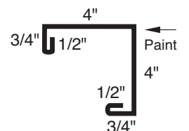
coin extérieur
