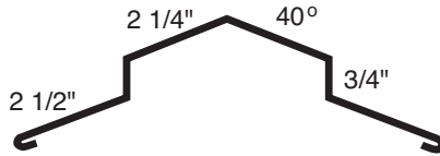
Faîtière boîte
