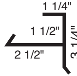
Solin de pignon en "F"
