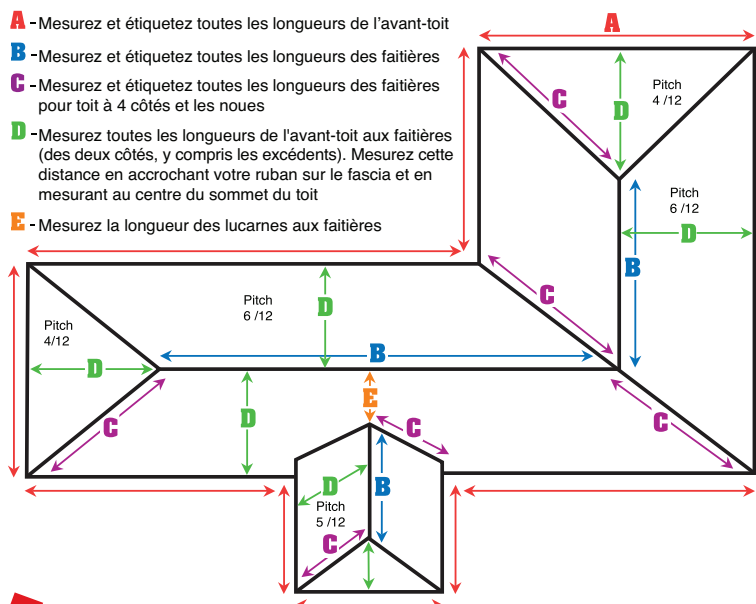
Toit à quatre versants
