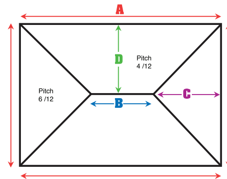
Toit en croupe
