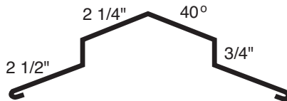
Box Cap
